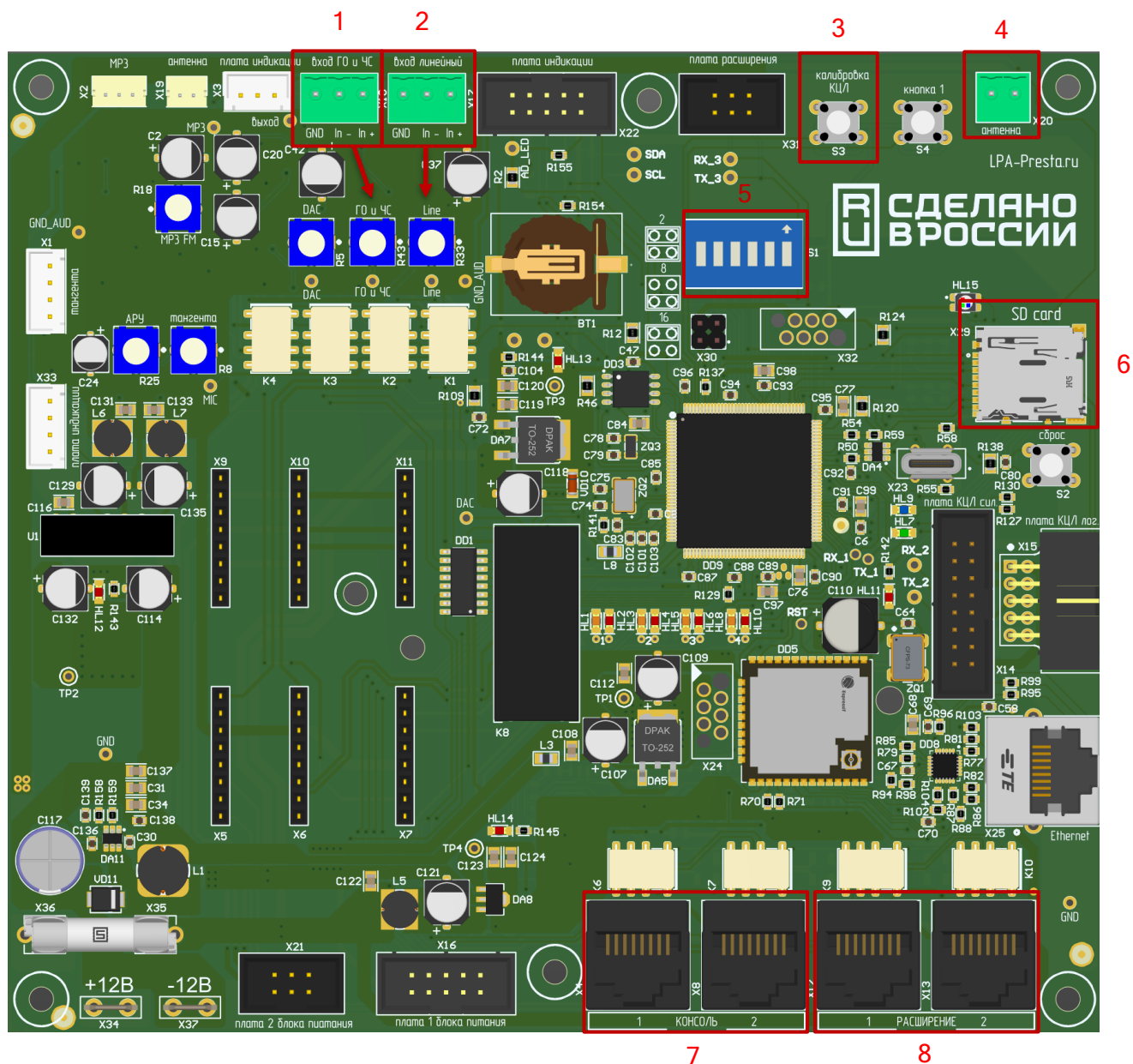
Рис. 2.5. LPA-Presta-2.ru плата управления
