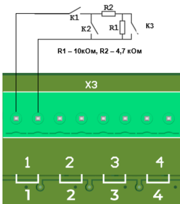
Рис. 3.3. Схема подключения внешних сигналов управления к LPA-Presta-2.ru с контролем целостности
