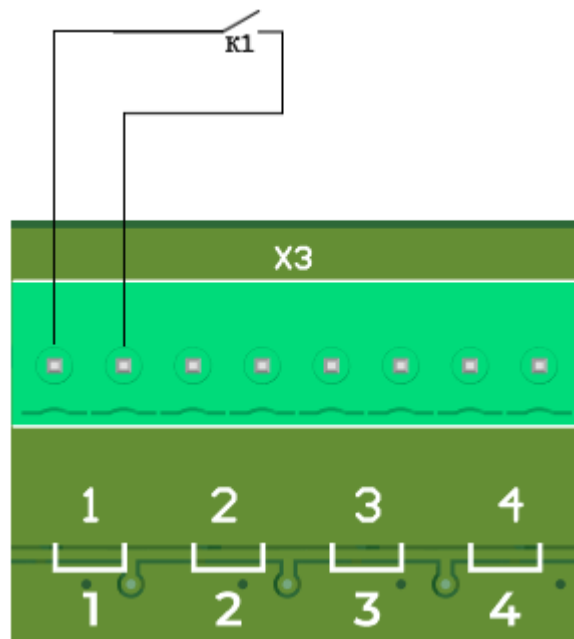
Рис. 3.4. Схема подключения внешних сигналов управления к LPA-Presta-2.ru без контроля целостности.
