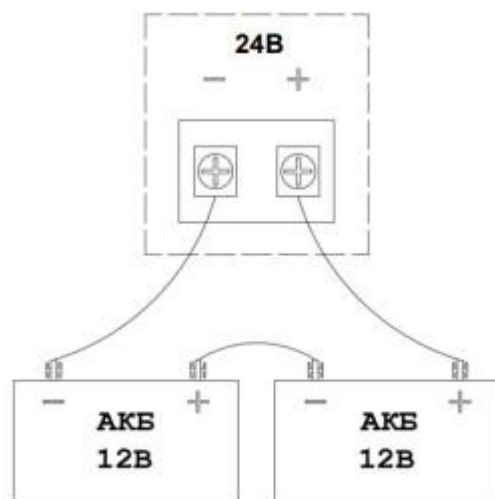
Рис. 3.1. Схема подключения АКБ к LPA-Presta-2.ru
