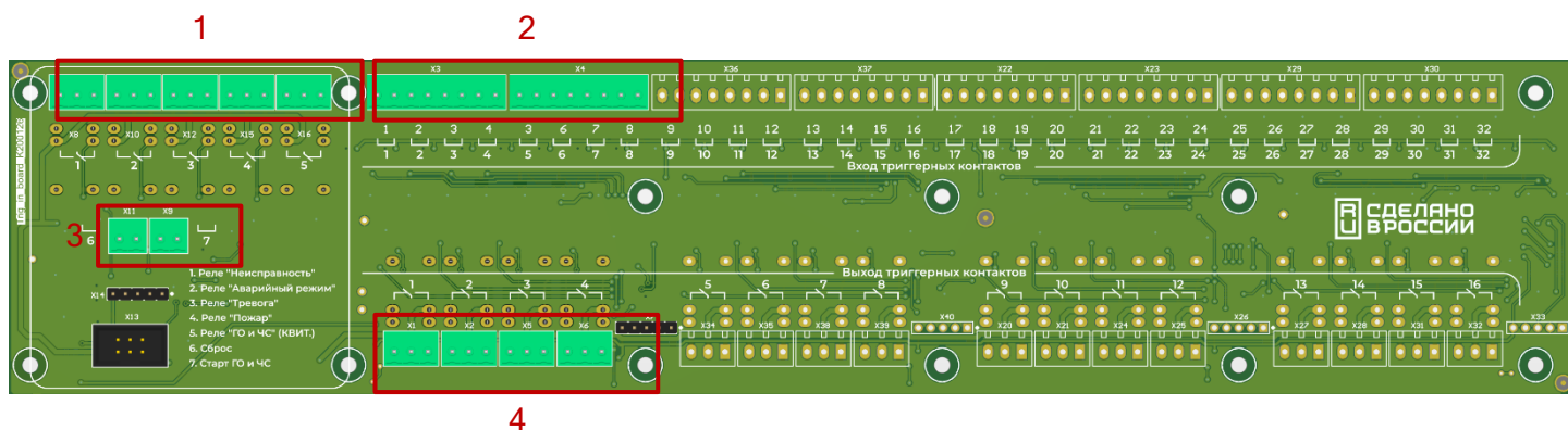
Рис. 2.2. LPA-Presta-2.ru плата расширения.
